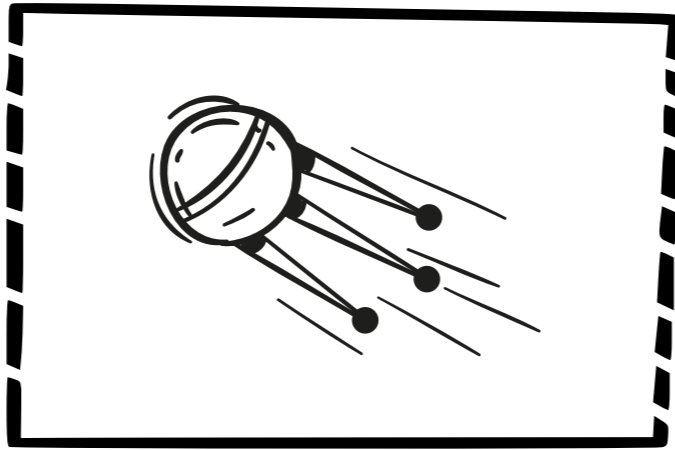
Искусственный спутник
