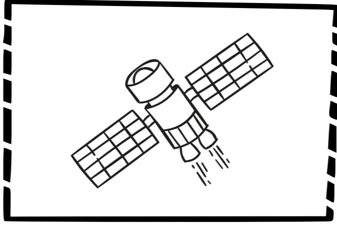
Космическая станция
