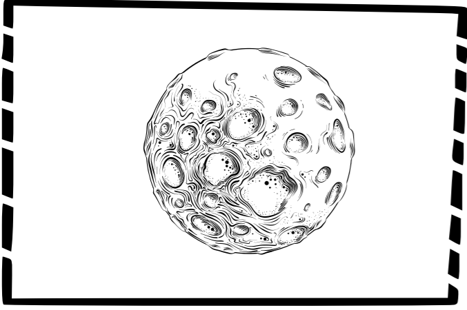
Естественный спутник
