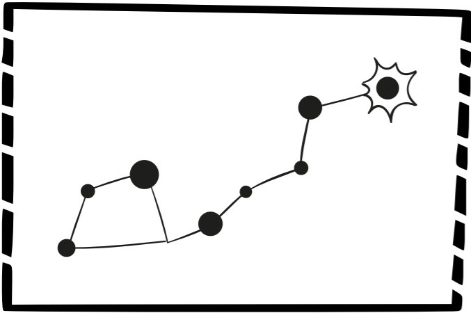
Созвездие
